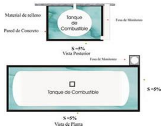
Figura No. 1 Tanques Soterrados
